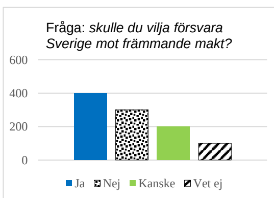
Figur 2. Hypotetiskt resultat från enkätfrågan i Figur 1.
