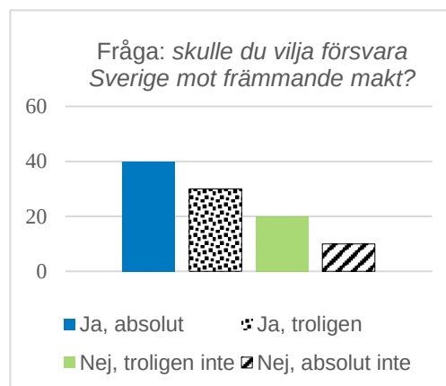
Figur 2. Hypotetiskt resultat från enkätfrågan i Figur 3. Figur 1. Hypotetiskt resultat från enkätfrågan i Figur 4.
