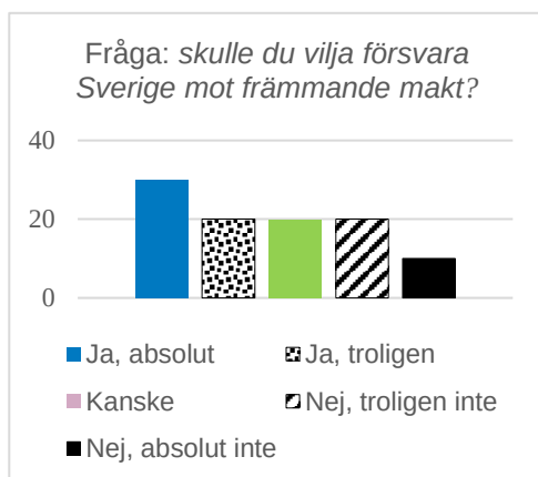
Figur 2. Hypotetiskt resultat från enkätfrågan i Figur 3. Figur 1. Hypotetiskt resultat från enkätfrågan i Figur 4.
